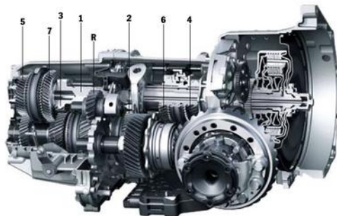
Porsche Doppelkupplung (PDK)
